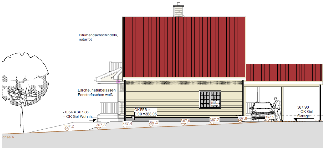
Südwestansicht Garage
