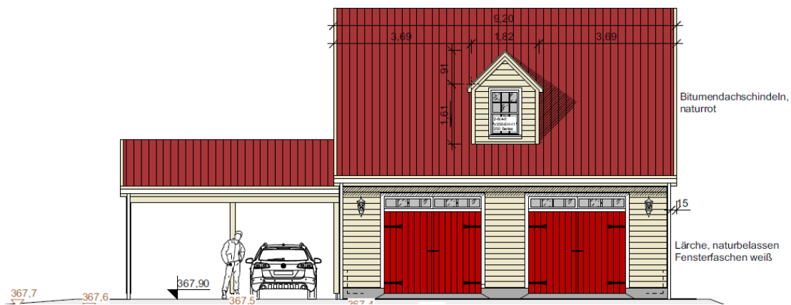
Südwestansicht Garage
